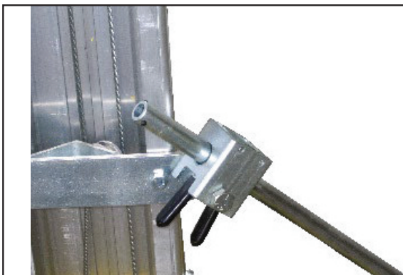
Arretierung der Ausleger sowohl in Arbeits- als auch in Lagerposition
